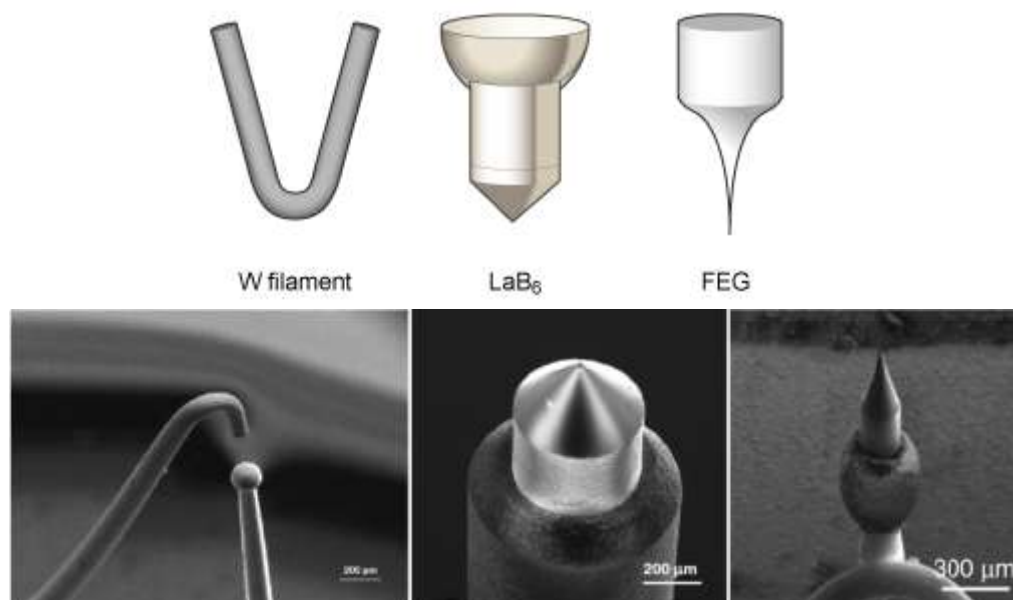
شکل ۳- تصویر فیلامان‌های تجاری رایج. ملاحظه می‌شود که فیلامان تنگستنی سنجاق سری به علت گرم شدن بیش از حد ذوب شده است که محل ذوب شدگی و قطره‌ی ذوب و منجمد شده قابل مشاهده هستند.
