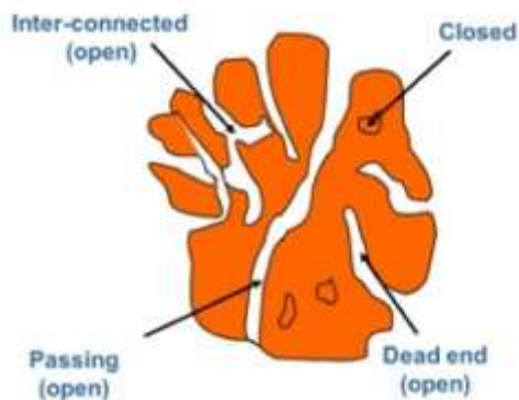
شکل ۲- نوع تخلخلها بر اساس شکل و موقعیت [۲].
