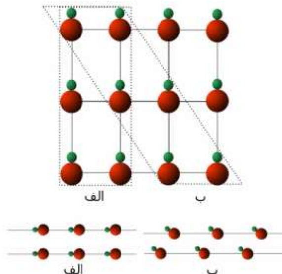
شکل ۲- فاصله صفحه‌ای متفاوت و آرایش مختلف اتم‌ها در دو صفحه از یک کریستال
