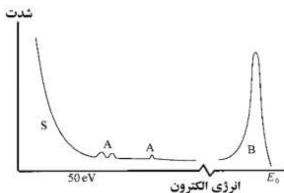
شکل ۶- طیف الکترونی که نشان‌دهنده فراوانی نسبی الکترون‌های ثانویه (S)، اوژه (A) و برگشتی (B) بر حسب انرژی الکترون است. توجه شود که مقیاس انرژی، پیوسته نیست؛ E ۰ به طور نمونه بسیار بیشتر از ۵۰ الکترون ولت است.
