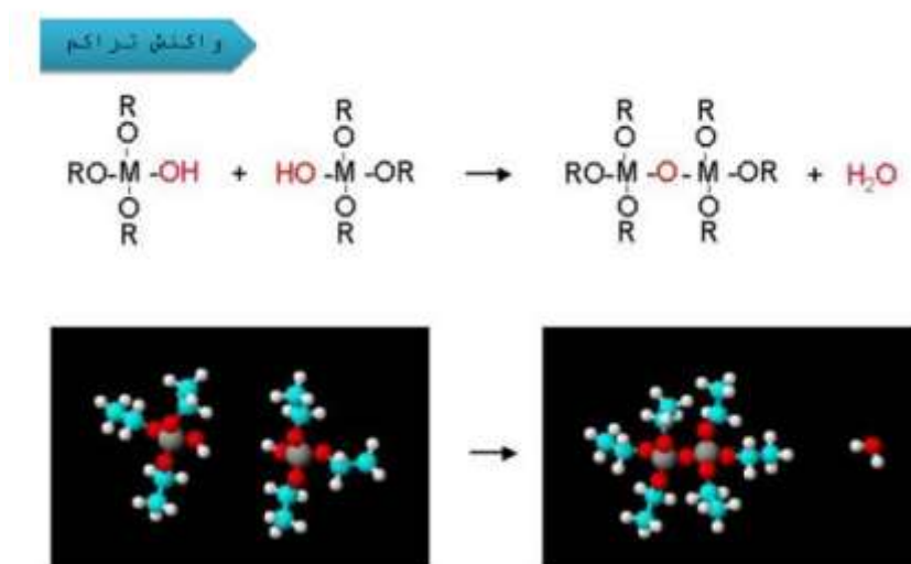
شکل ۴- تصویر مدل سه بعدی مربوط به واکنش تراکم
