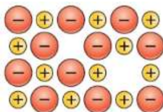
شکل ۶- نمایش عیب شاتکی
