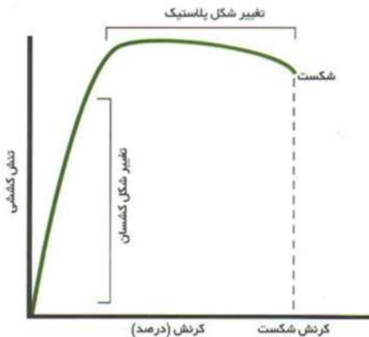
شکل ۴: نمودار تنش-گرنش بدست آمده از آزمون کشش یک نمونه
