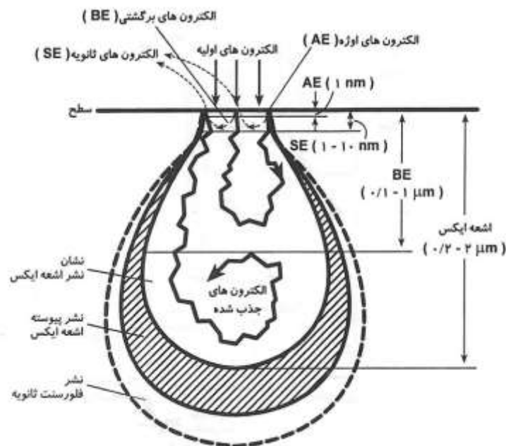
شکل ۸- عمق نفوذ پدیده‌های مختلف ناشی از برهمکنش پرتوی الکترونی و نمونه
