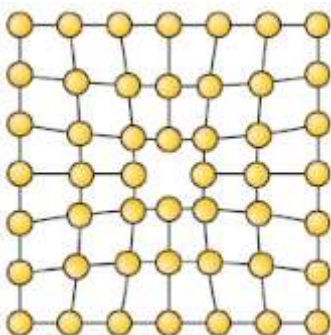
شکل ۲- نمایش جای خالی در یک ساختار بلوری [۲]
